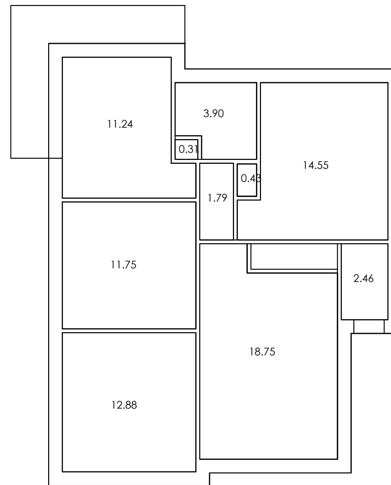
PLANTA ALTA
